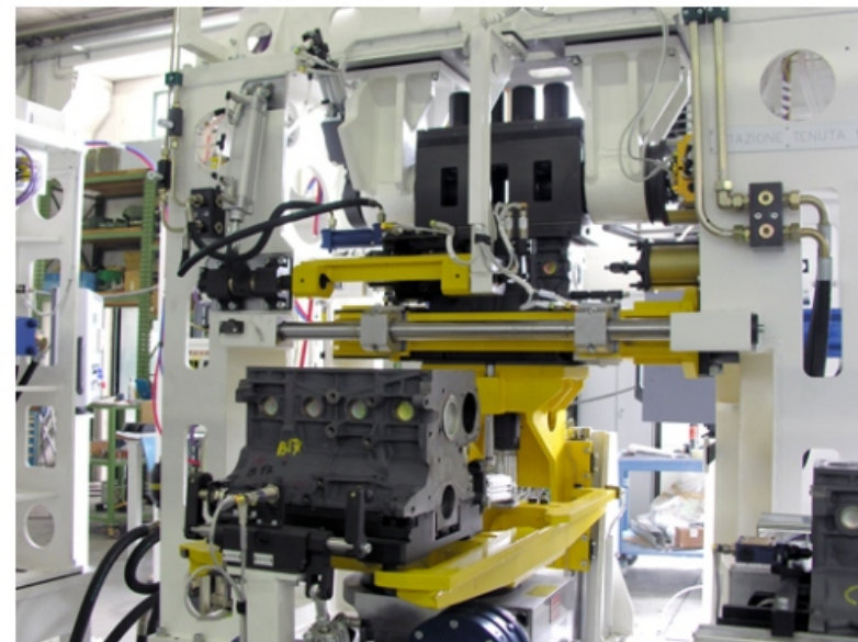
Dispositivo estandarizado para LEAK Test
